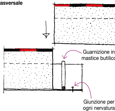
Giunzione trasversale
